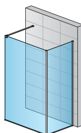
GLA (5) + WPE + D40
