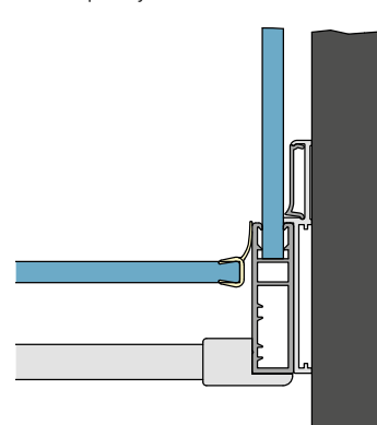
Detail A půdorys:
