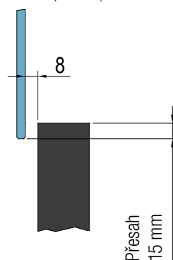
Detail A pohled zředu:
