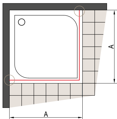
Obr. 1 Dveře, rohový vstup, čtvrtkruh
