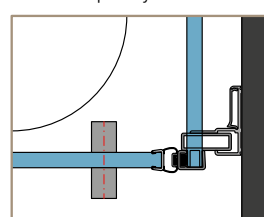
Detail A - půdorys
