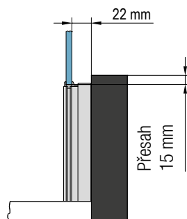
Detail A pohled zředu:
