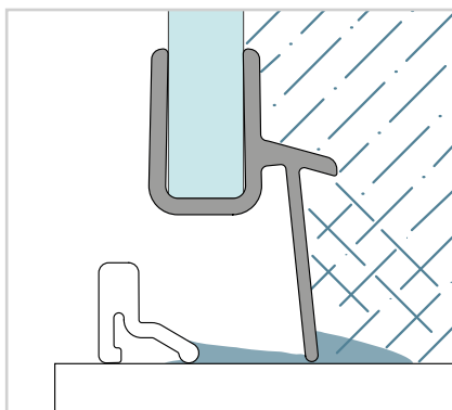
Částečně rámové zástěny s prahovou lištou
