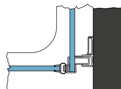
Detail A půdorys:
