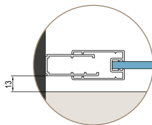
Obr. 1 Dveře, rohový vstup, čtvrtkruh
