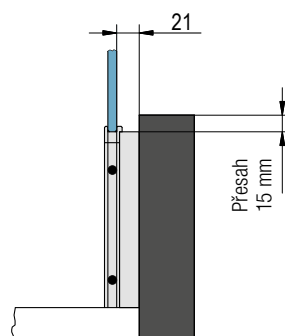
Detail A - pohled zepředu
