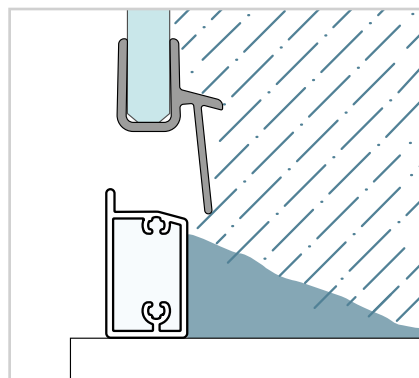
Rámové zástěny s rámovými profily
