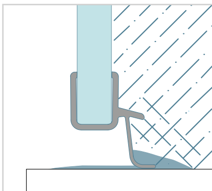
Bezrámové zástěny bez prahové lišty
