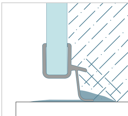
Bezrámové zástěny bez prahové lišty
