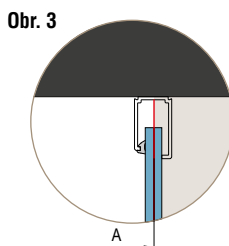
Pevná stěna v 90°
