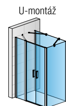
U-montáž D22T32 + D22F1 + D22F3 + D22EV1 + D22EV2
