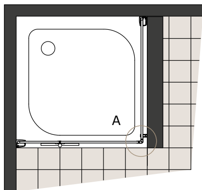
Detail A - pohled zředu
