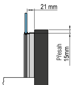
Detail A - pohled zepředu
