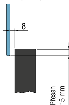
Detail A pohled zpredu:
