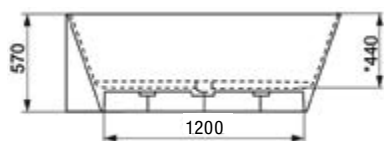
INSTALLATION DROITE
