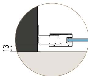
Fig. 1 Portes coulissantes D20S2, D20SE2 & D20SR
