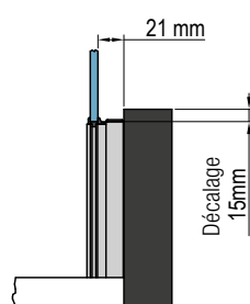
Détail A - vue de face
