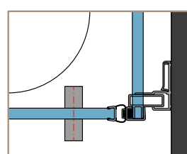
Détail A - vue du dessus
