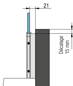
Détail A vue de face :
