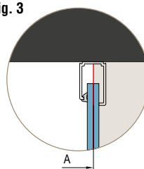
Paroi fixe à 90°
