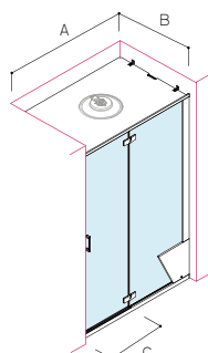
INSTALLATION EN NICHE
