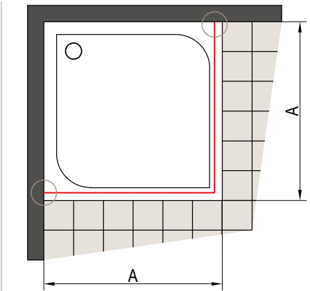
A | Dimension mesurée du mur, carrelage posé, au bord extérieur du receveur.
