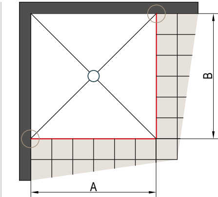
A-B | Dimension mesurée du mur, carrelage posé, à la position réelle de la paroi
