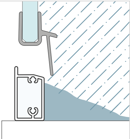
Parois de douche avec profilé de cadre
