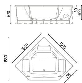
Positionnement conseillé de la baignoire
