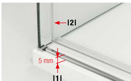
Porte coulissante
