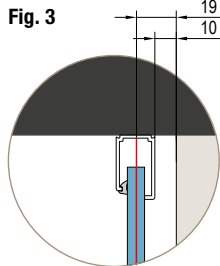
Paroi fixe à 90°
