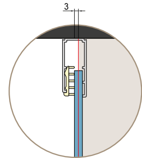
A-B | Dimension mesurée du mur, carrelage posé, à la position réelle de la paroi
