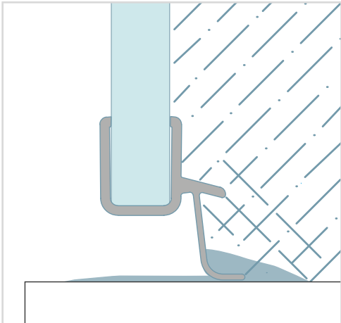
Parois de douche sans cadre et sans barre de seuil
