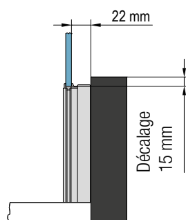
Détail A vue de face :
