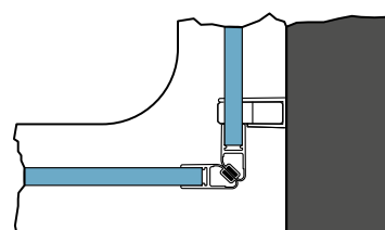
Détail A vue de dessus :
