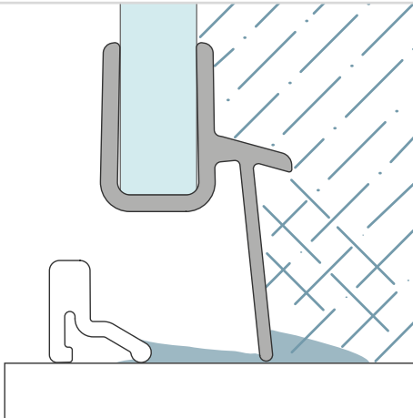
Parois de douche avec profilés et profilé de seuil moyen
