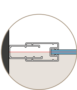
A-B | Dimension mesurée du mur, carrelage posé, à la position réelle de la paroi
