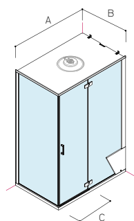
INSTALLATION EN ANGLE
