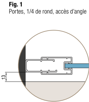
A | Dimension mesurée du mur, carrelage posé, au bord extérieur du receveur.
