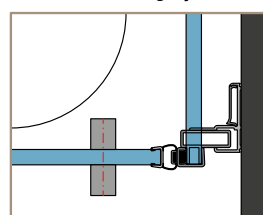
Detal A - widok z góry:
