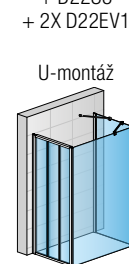
2X D22F1 + D22S3 + 2X D22EV1
