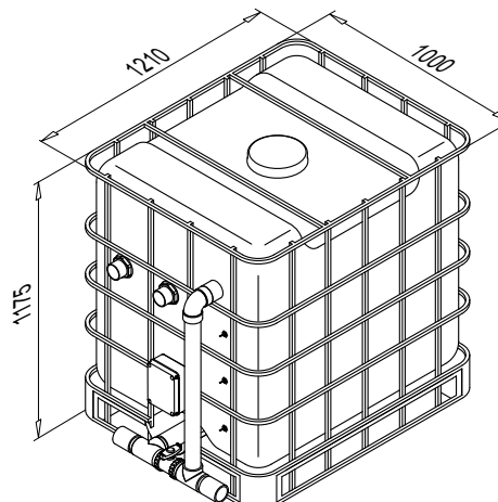
VASCA DI COMPENSO COMPENSATION TANK KOMPENSATIONSBECKEN CUBA DE COMPENSACIÓN VASQUE DE COMPENSATION
